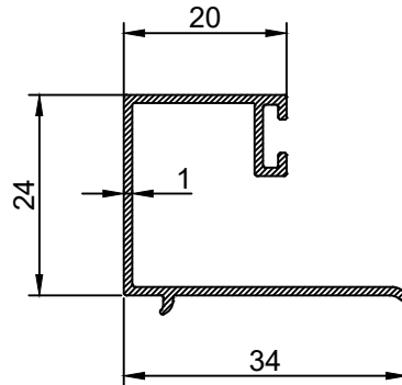
ER 7193 0,255 Kg/m 29mm.Cama Göre Çıta Glazing With 29mm.Gap
