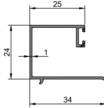
ER 7192 0,268 Kg/m 24mm.Cama Göre Çıta Glazing With 24mm.Gap
