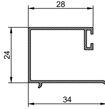
ER 7176 0,279 Kg/m 20mm.Cama Göre Çıta Glazing With 20mm.Gap
